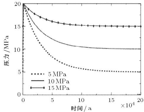
图 3 不同上边界压力下 CO 2 压力消散
