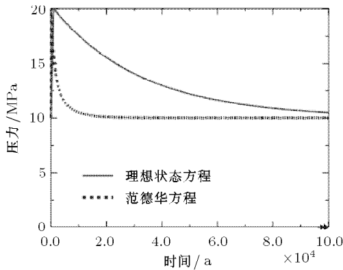
图 5 不同气体状态方程时 CO 2 压力消散
