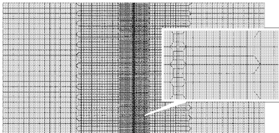
图 2 含井地层网格剖分图
