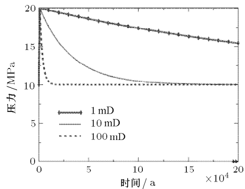
图 4 不同渗透系数时 CO 2 压力消散
