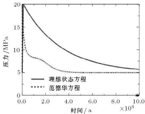
图 6 不同气体状态方程时 CO 2 压力消散
