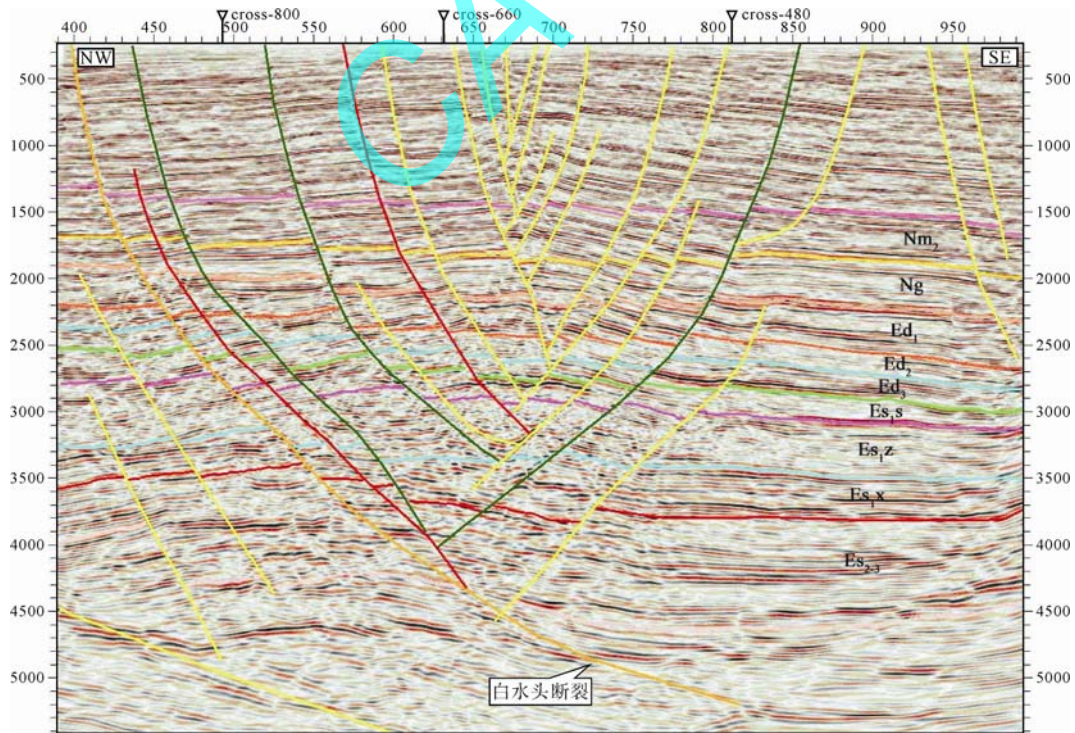
图 7 白东构造带 Inline2680 测线地震剖面(测线位置见图 1)
