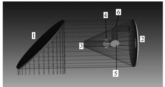
图 6 偏振保持光路在接收系统中的应用
