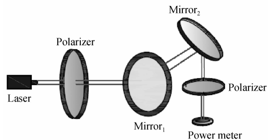
图4 偏振保持设计光路
