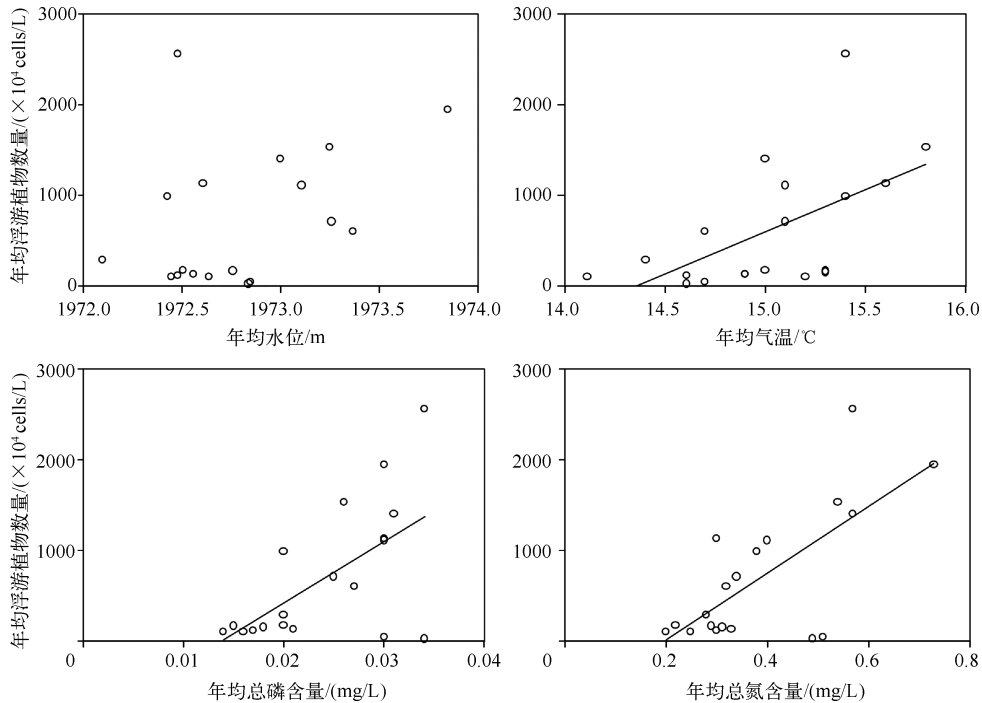
图2 1980—2009年浮游植物数量与洱海水位、气温、水体氮磷的关系
