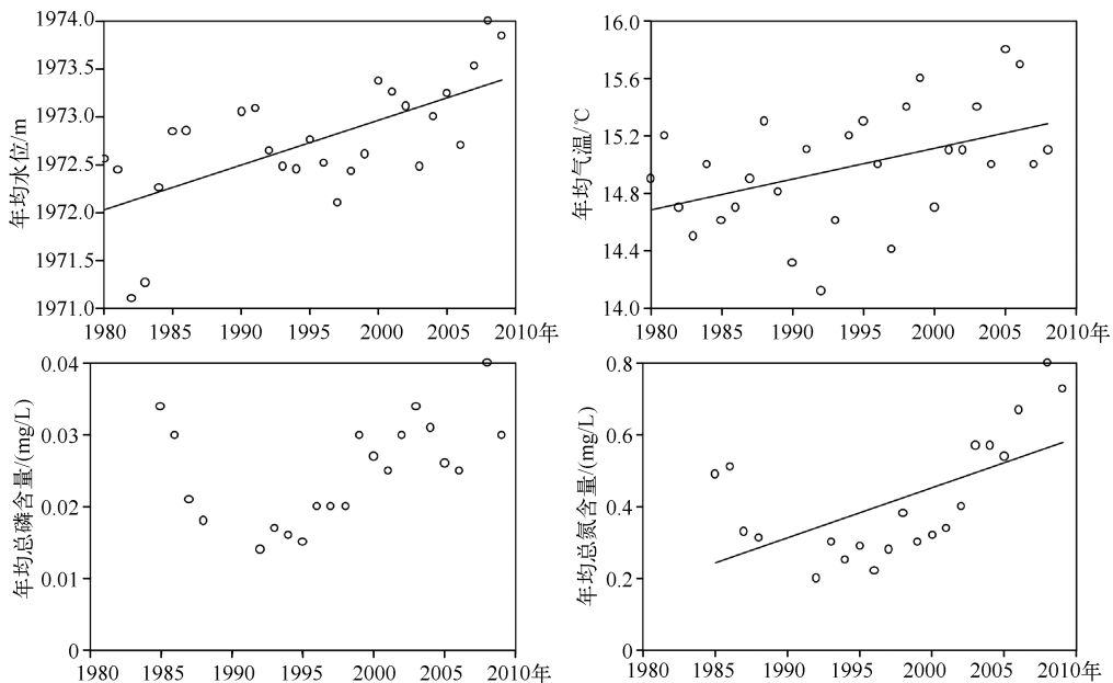
图 1 1980—2009 年洱海年均水位、气温、水体总磷、总氮变化
