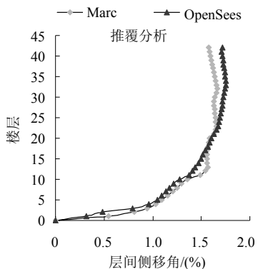
图 9 静力推覆层间位移角分布图 Fig.9 Distribution of drift angle
