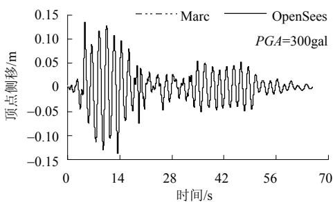
(b) ChiChi 波 300gal 动力时程分析结果
