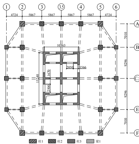
图 6 结构平面图
