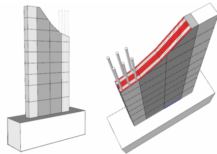
图 3 分层壳模拟剪力墙单元划分示意图
