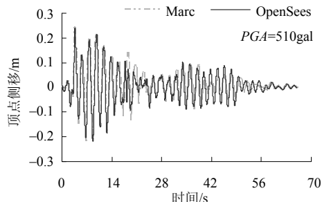
(c) ChiChi 波 510gal 动力时程分析结果
