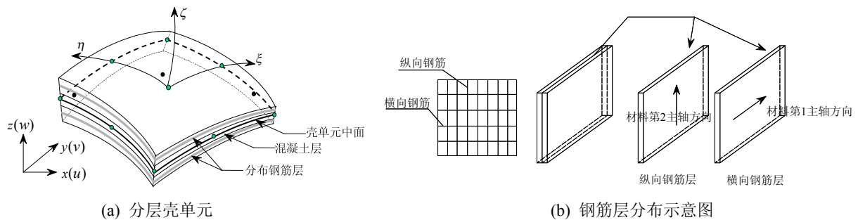
图 1 分层壳单元示意图 Fig.1 Multi-layer shell element
