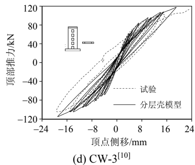
图 4 试件顶点力-位移滞回曲线
