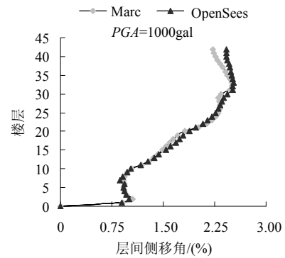
(d) Northridge 波结构层间位移角包络图对比
