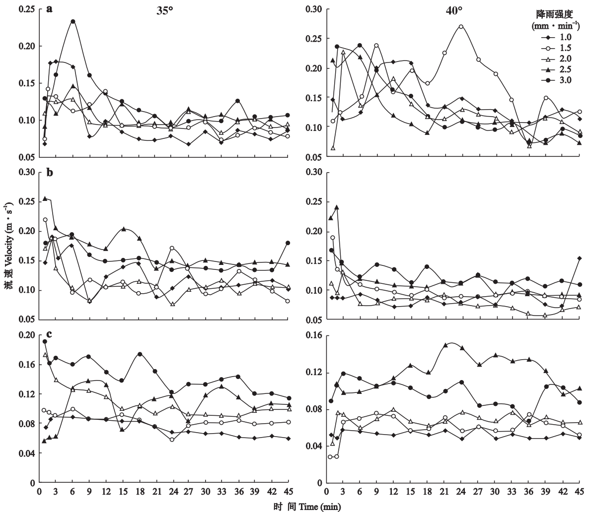
图2 弃土弃渣体径流流速随时间的变化
