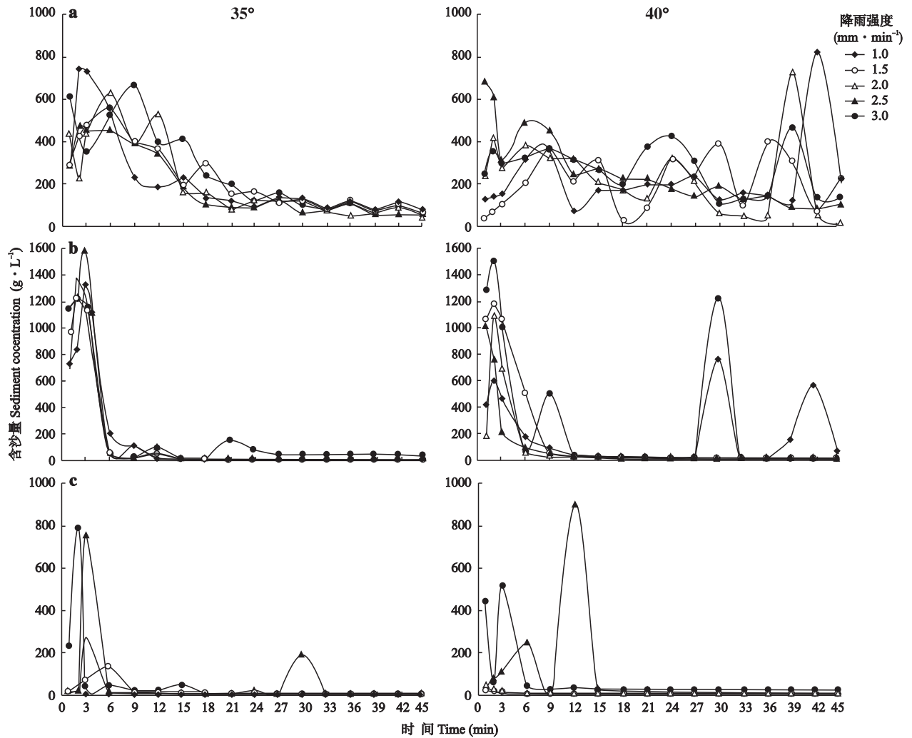
图4 弃土弃渣体含沙量随时间的变化
