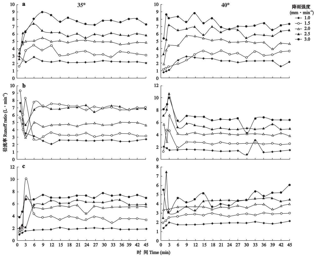
图3 弃土弃渣体径流率随时间的变化
