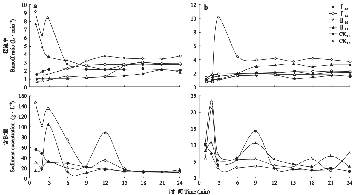
图 5 弃渣防护体径流率和含沙量随时间的变化
