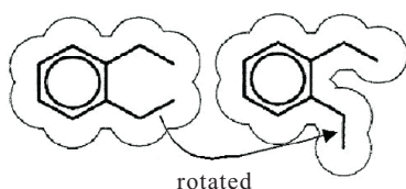
图 1 同一种分子的不同低能形状
