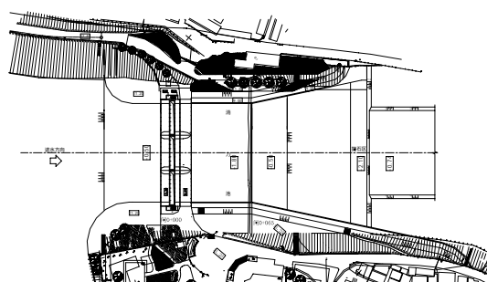
图1 补充方案 平面布置
