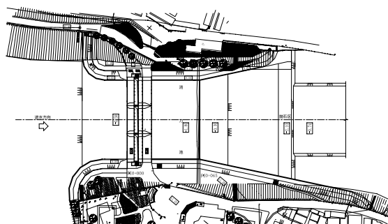
图1 补充方案 平面布置
