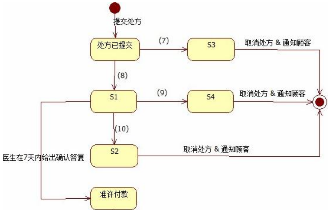
图 3-2 状态图
