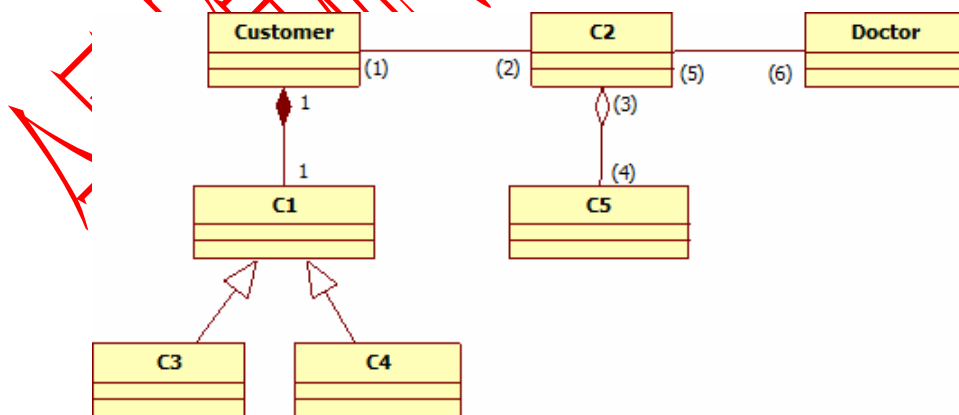
图 3-1 类图
