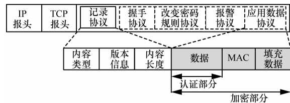
图 4 SSL 安全协议数据封装格式
