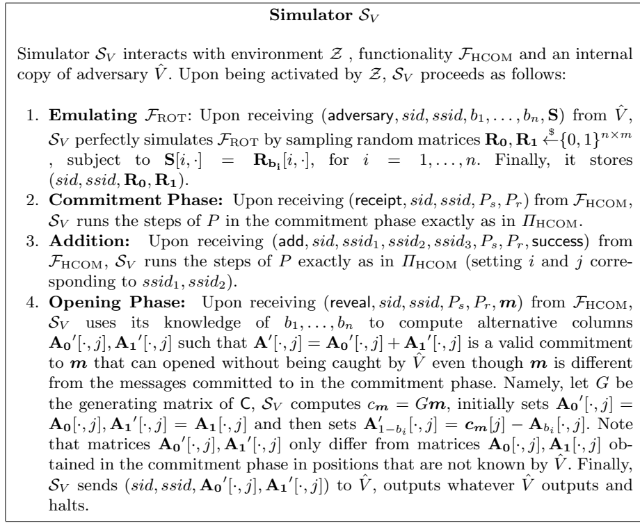
Fig. 6. Simulator \mathcal{S}_V
