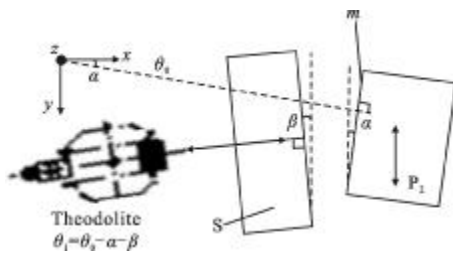
图 2 直角棱镜及检偏器光轴偏离角
