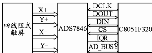
图 1 接口连接图
