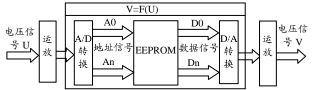
图 1 操纵台输出电压曲线修正框图
