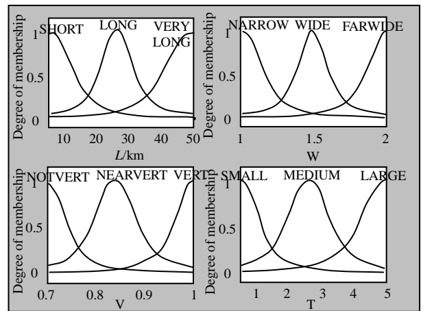
图 7 输入隶属度函数
