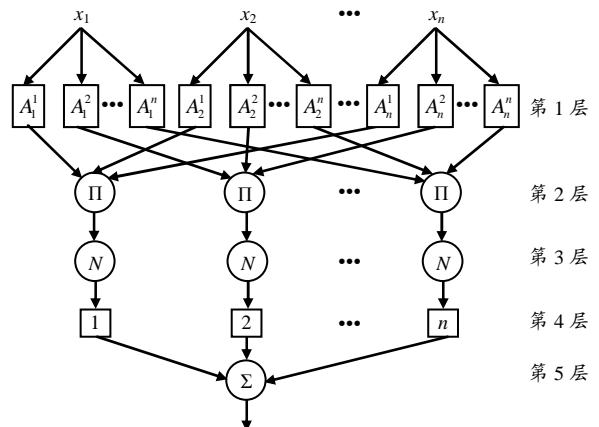
图 4 ANFIS 系统结构图
